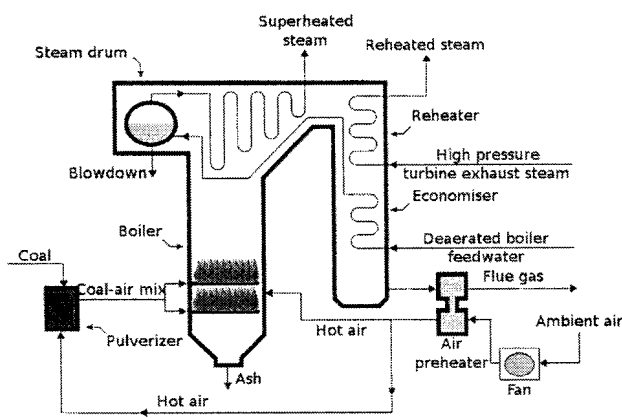
หม้อไอน้ำแบบที่-2
