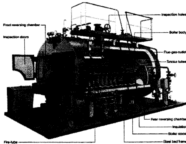
หม้อไอน้ำแบบที่-1
