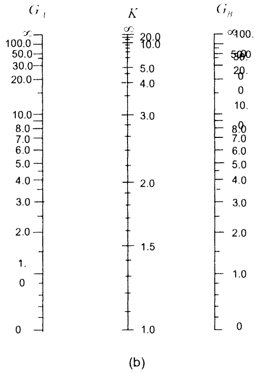
แบบจำลองของเสาในโครงข้อแข็งที่ยึดรั้งด้านข้าง และแผนภาพ Alignment
